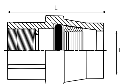
Sivuliitin
